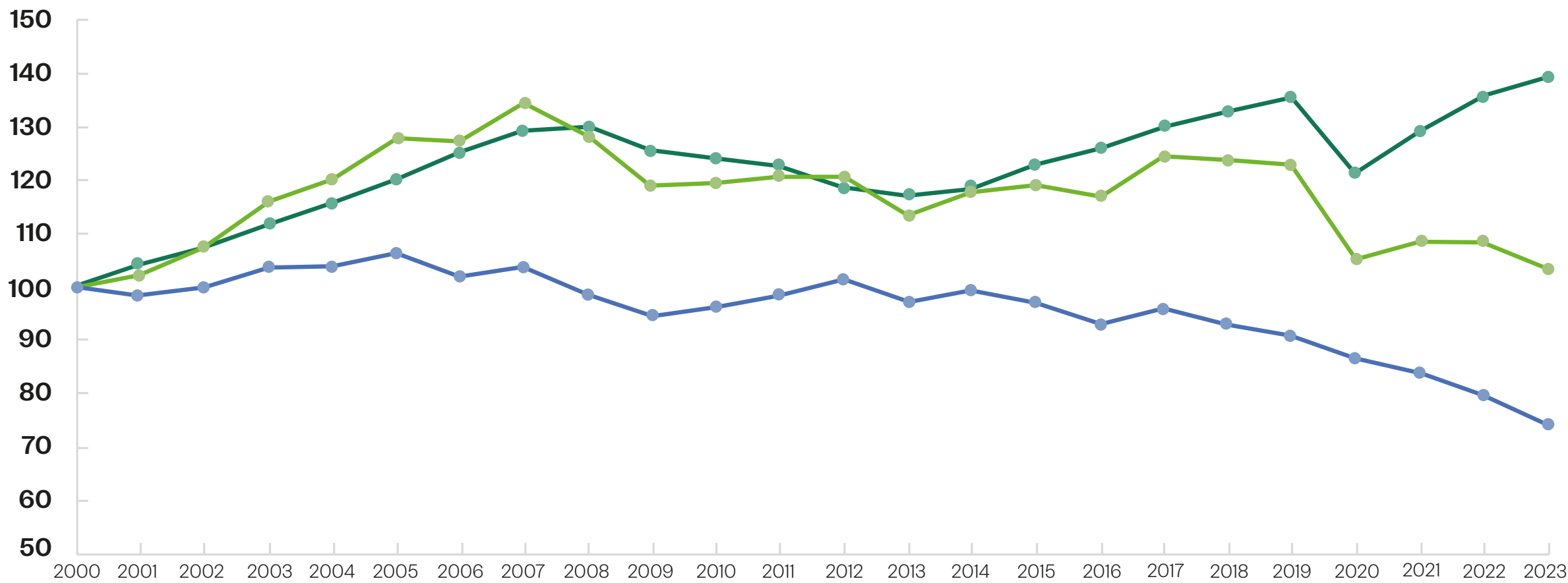
Índice 2000=100
