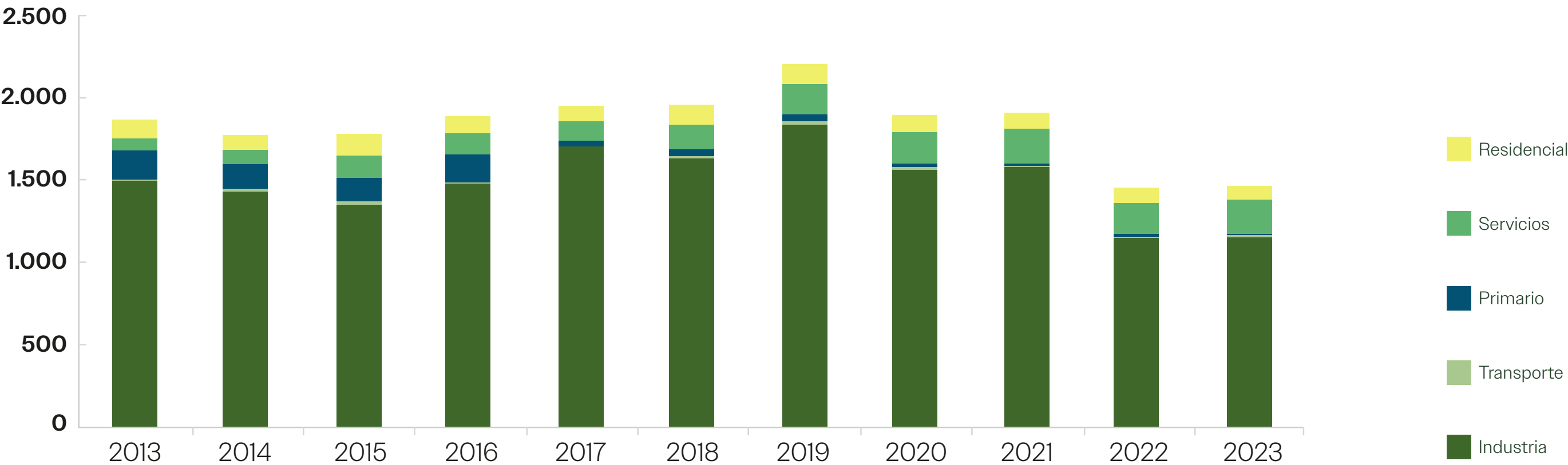
Unidad: ktep
