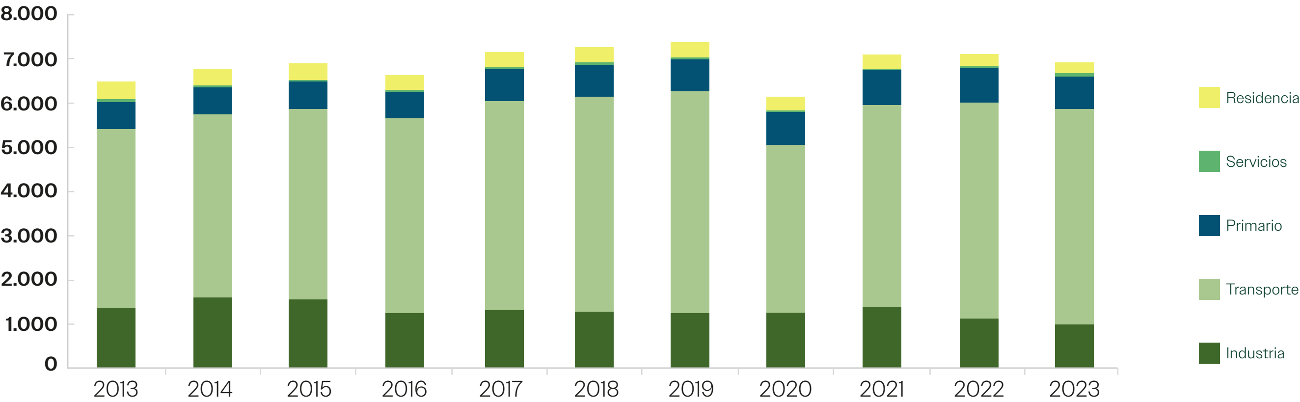
Unidad: ktep
