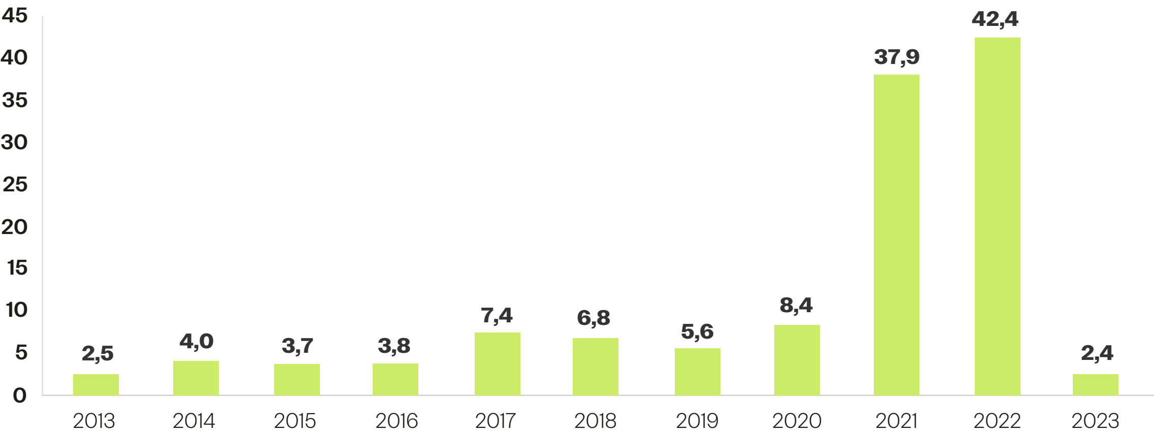
Unidad: ktep
