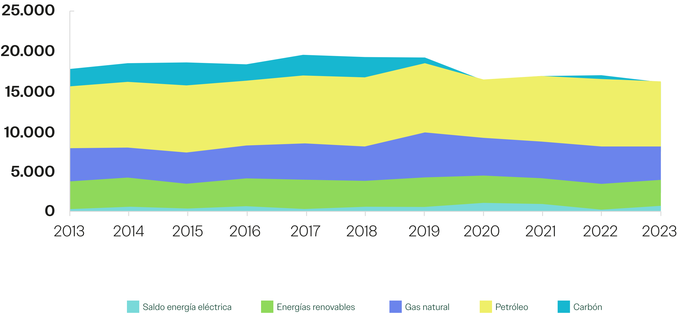
Unidad: ktep
